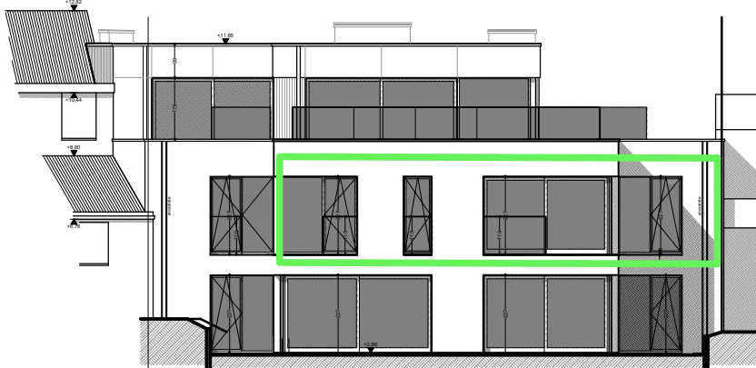
Façade arrière 1:200 [cm] Situation projetée
