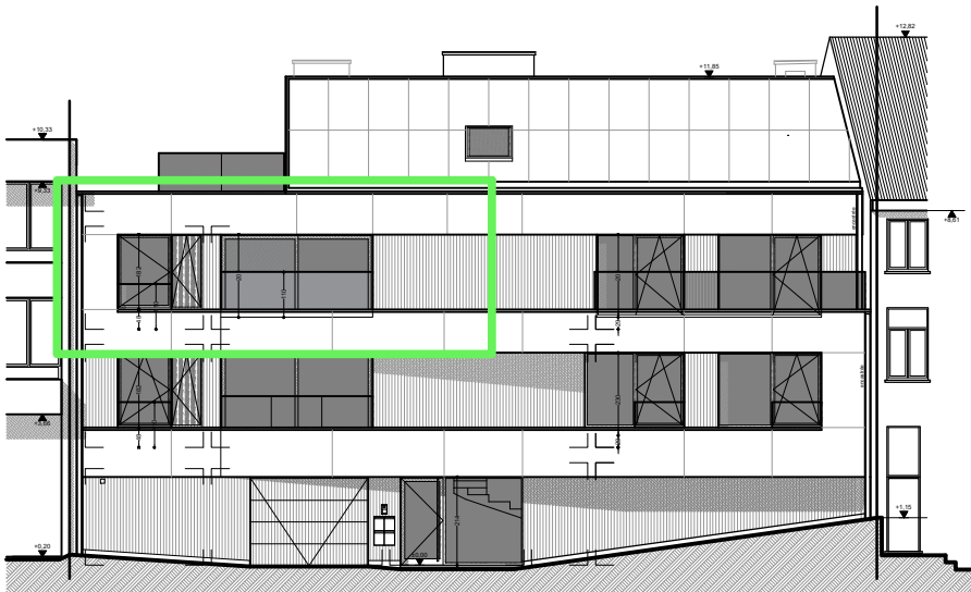
Façade avant Situation projetée 1:200 [cm]
